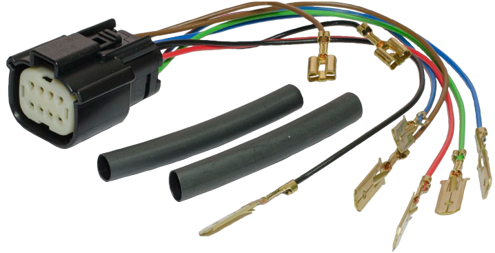
Fig. 9.3 : câble adaptateur SingleViu WWG
