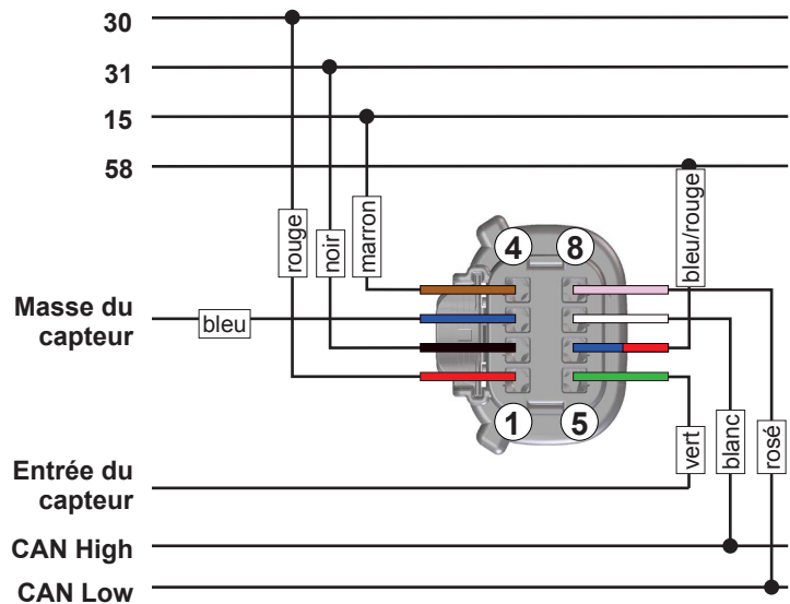
Fig. 3.2 : Schéma de câblage connecteur 8 voies
