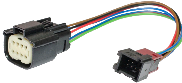
Fig. 9.1 : câble adaptateur SingleViu Viewline 8 broches
