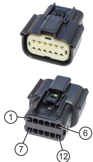
Fig. 6.5 : connecteur MOLEX 12 broches
