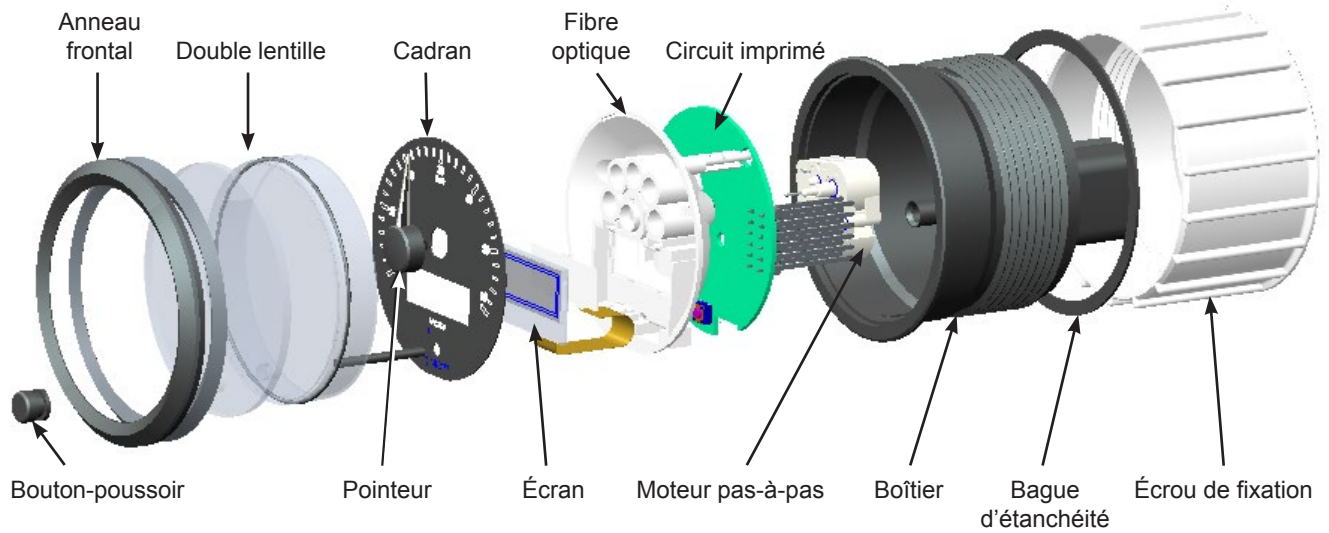
Fig. 4.1 : structure d'un instrument SingleViu.
