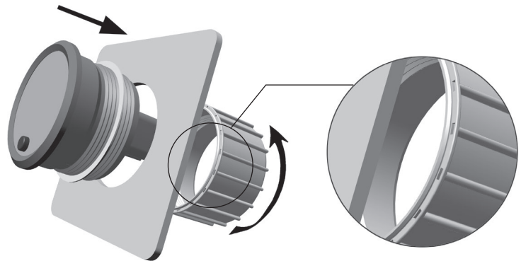
Fig. 6.6 : insérer l'instrument.
