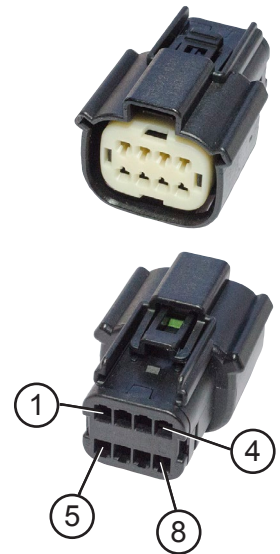
Fig. 6.4 : connecteur MOLEX 8 broches
