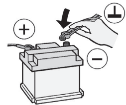
Fig. 6.8 : raccorder la batterie.
