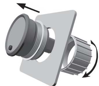
Fig. 11.4 : retirer l'instrument
