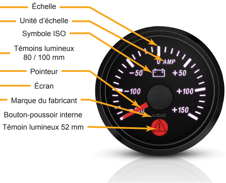
Fig. 4.3 : éléments du cadran 52 mm
